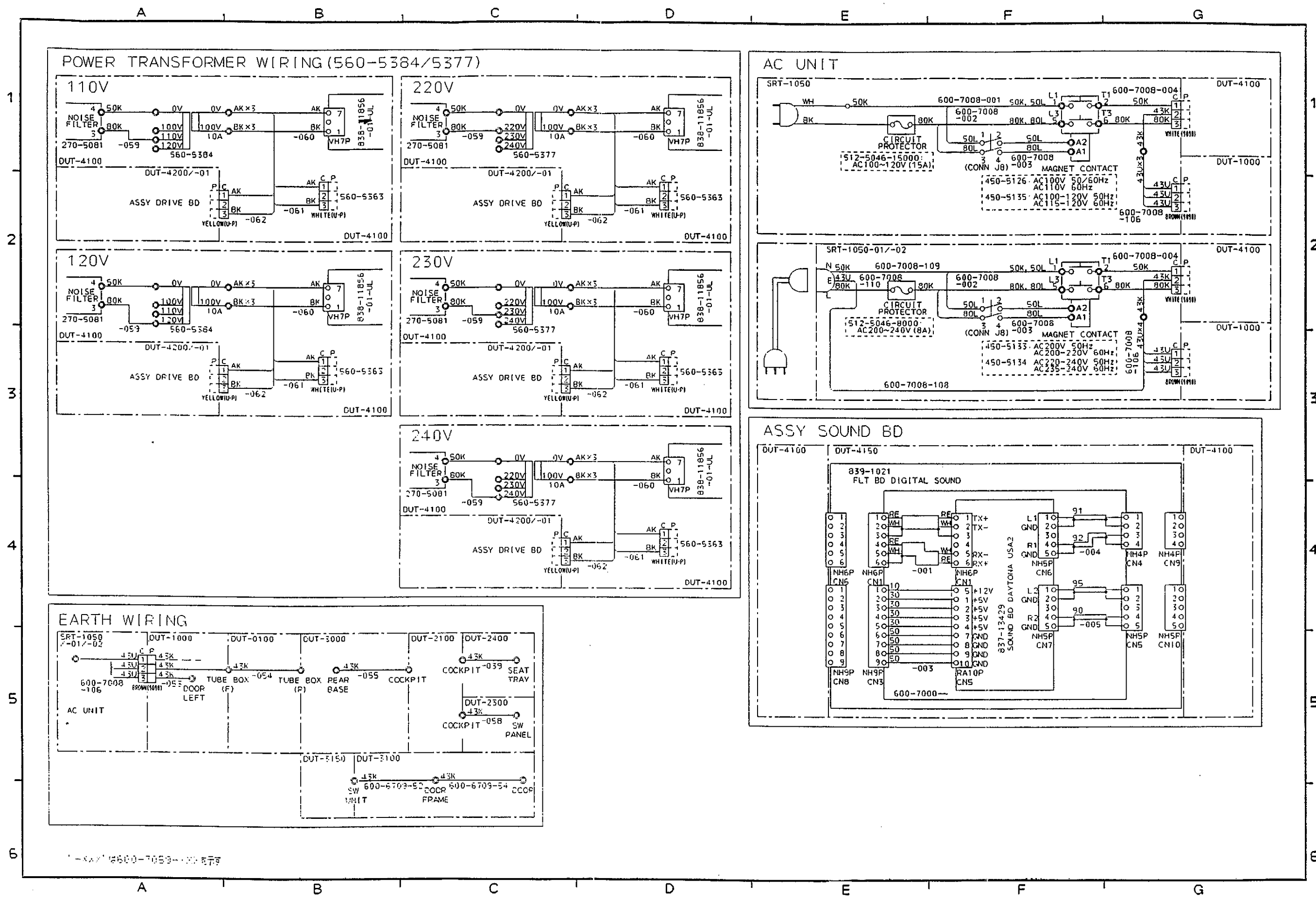
24. WIRING DIAGRAM (D-3/3)
