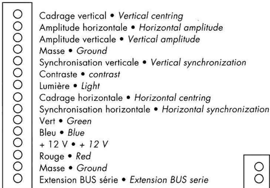
J1 Connecteur du module de réglage Control module connector
