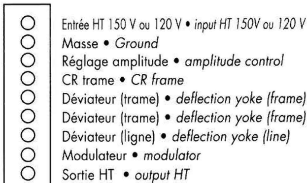
Connecteur Est ouest East west connector
