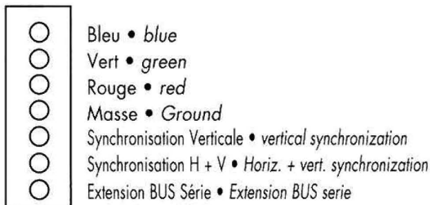
J2 Entrée signaux RVB + synchro Signals input RVB + synchro
