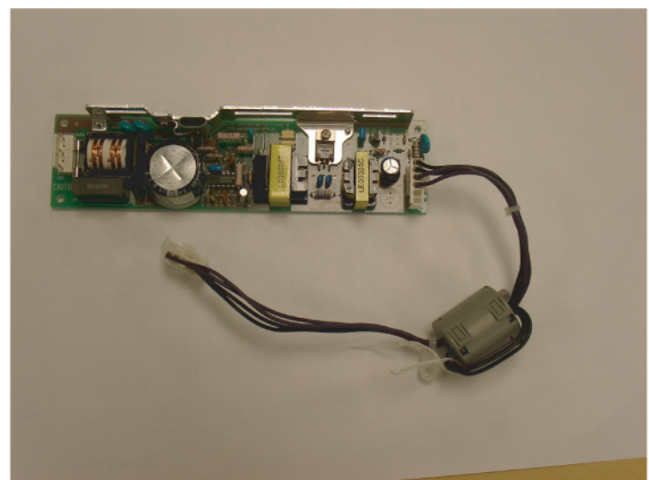
400-5421-05024 POWER SUPPLY(COSEL)
